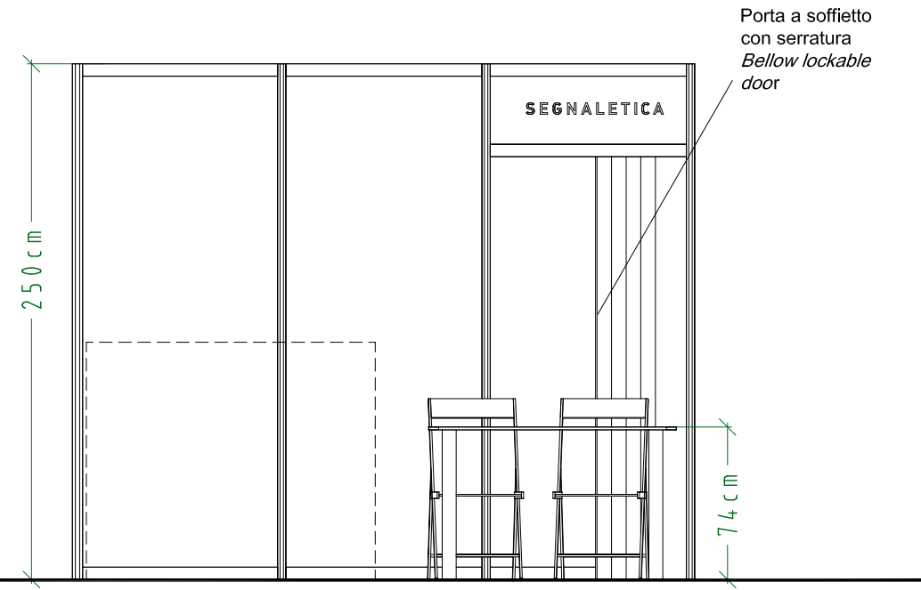
PROSPETTO/FRONT ELEVATION
