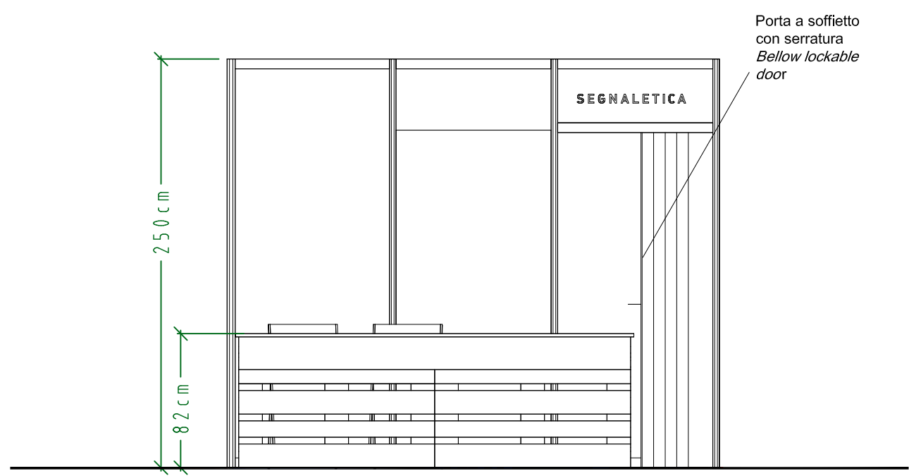
PROSPETTO/FRONT ELEVATION
